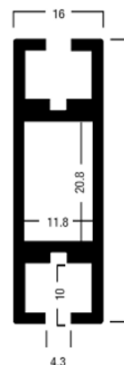
przekrój łącznika
